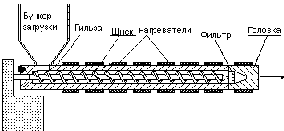
Рис1. Упрощенная схема экструдера
